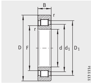
SL1923 Stützlager
