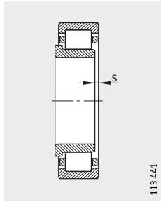
1) Axialer Verschiebeweg „s“ für NJ
