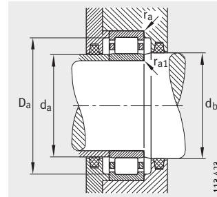
Anschlussmaße für NU
