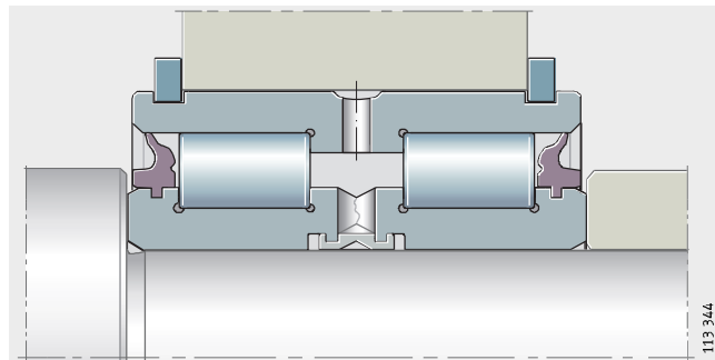
Bild 1 axial fixierter Außen- und Innenring
