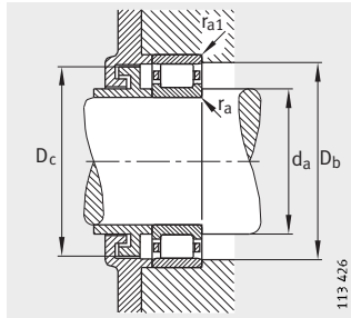
Anschlussmaße für N
