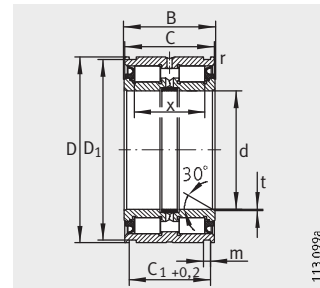
SL0450...-PP SL04...-PP
