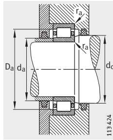
Anschlussmaße für NJ
