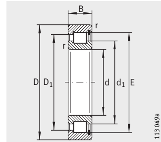
SL1818, SL1829, SL1830, SL1822 Stützlager
