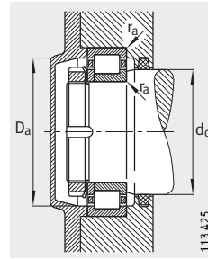
Anschlussmaße für NUP
