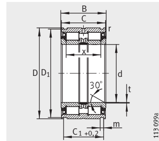
SL0450...-PP SL04...-PP
