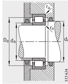
Anschlussmaße für NJ
