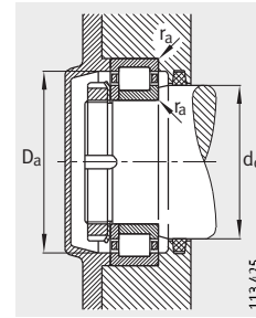
Anschlussmaße für NUP
