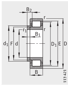
NJ und HJ
