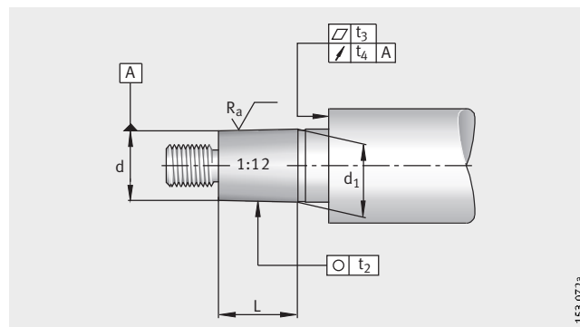
Bild 1 Ausführung der Welle
