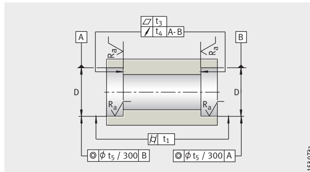
Bild 2 Ausführung des Gehäuses
