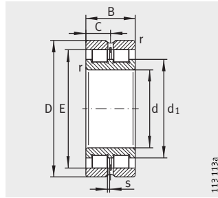
SL0248, SL0249 Loslager
