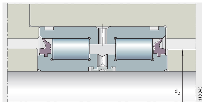
Bild 2 Unterstützung der Dichtringe
