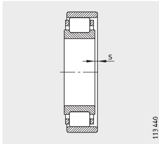
1) Axialer Verschiebeweg „s“ für N und NU
