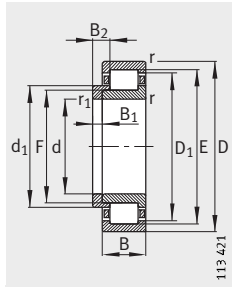
NJ und HJ
