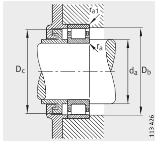
Anschlussmaße für N248-E-M1: D_{b \min} = 396 \text{ mm} D_{c \max} = 390 \text{ mm}
