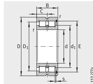
SL1850 Stützlager
