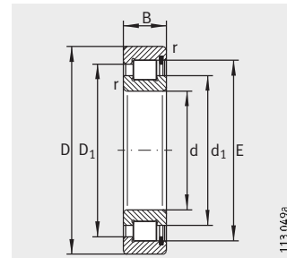
SL1829, SL1830, SL1822 Stützlager
